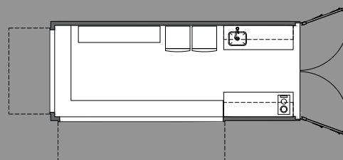
PLANTA ARQUITECTURA
