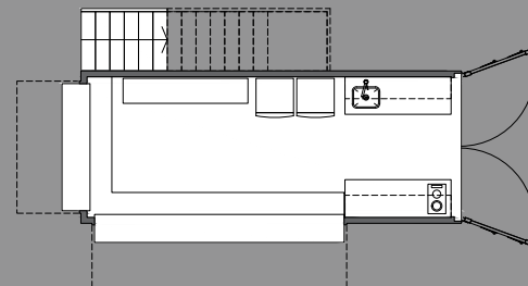
PLANTA BAJA
